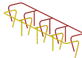
Лабиринт СКК 064 Размер 4030*1120*700
