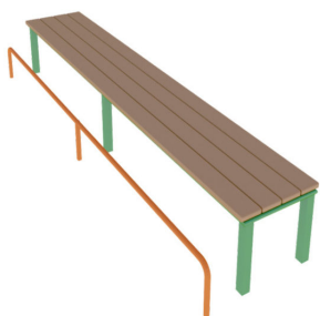
Скамья гимнастическая с упором для ног СКС 036 Размер 3000*805*450
