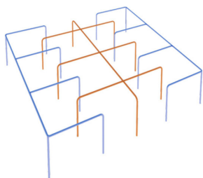
Лабиринт большой СКК 047 Размер 3180*1380*700
