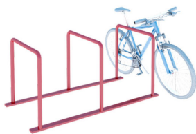
Велопарковка 2 СКС 072 Размер 800*1700*800
