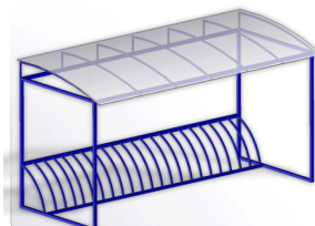
Велопарковка СКС 003 Размер 3000*1800*2200
