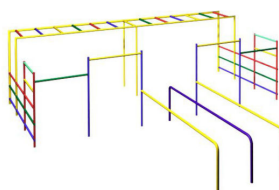
Спортивный комплекс 3 СКС 075 Размер 5300*5000*2300
