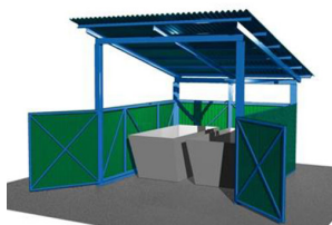
Навес для 1 мусорного бункера 8м3 СКП 114
